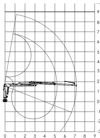
Reichweitendiagramm OL 7450 SG/P
